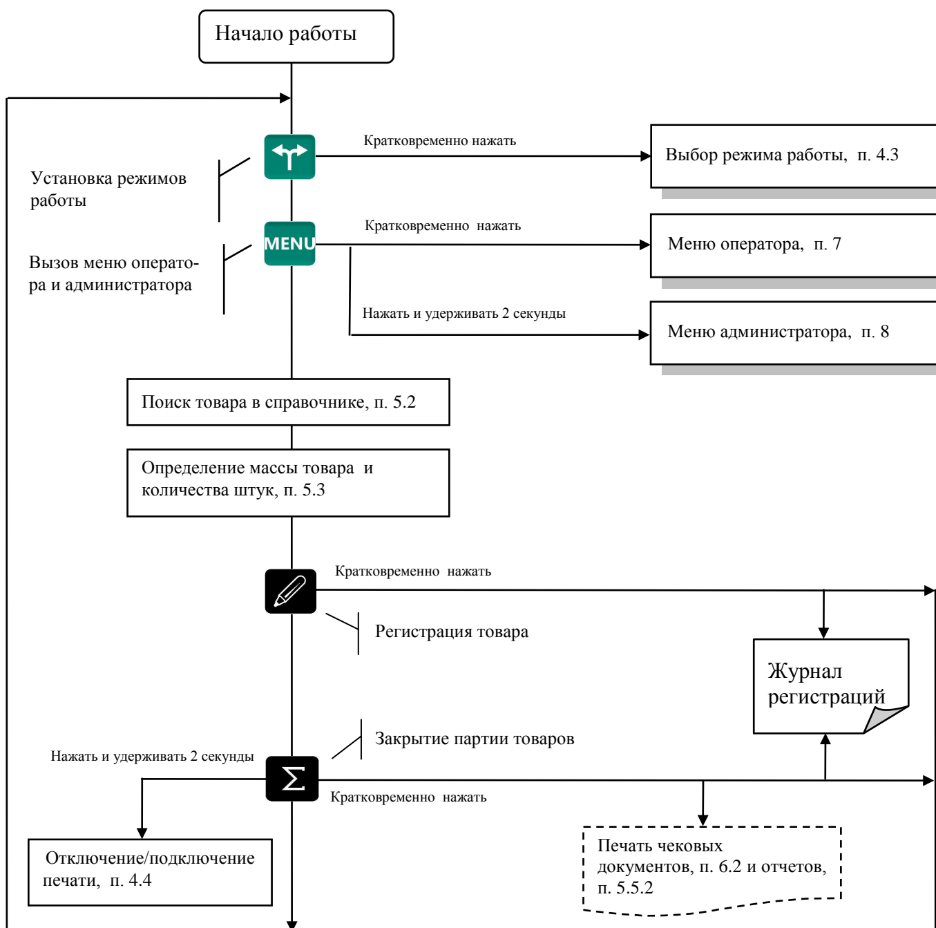
Рис. 3.1 - Схема работы терминала RC
