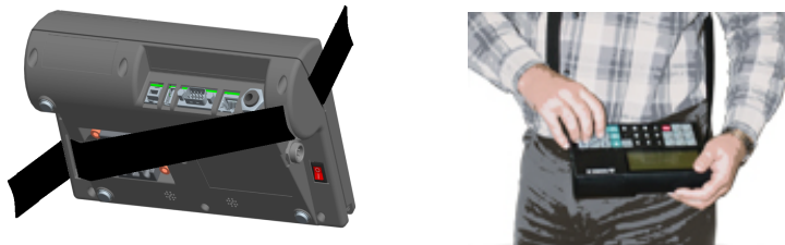
Рис. 2.3 - Крепление ремня для переноски терминала РС
